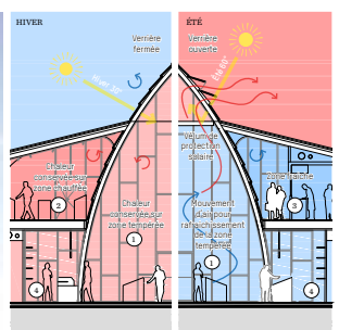
Détail sur la verrière - Principes bioclimatiques - 50e
