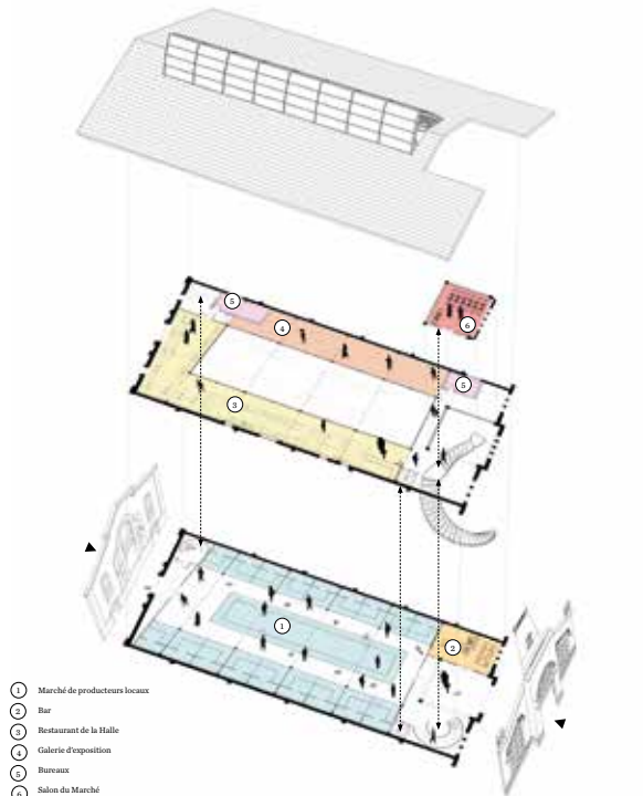
Principe projet - axonométrie des niveaux
