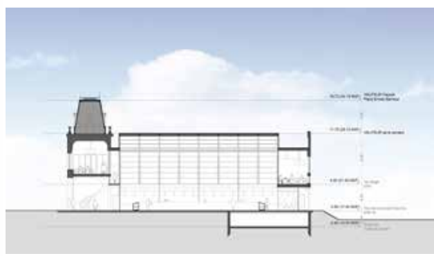
Coupe en long DD' - 200e
