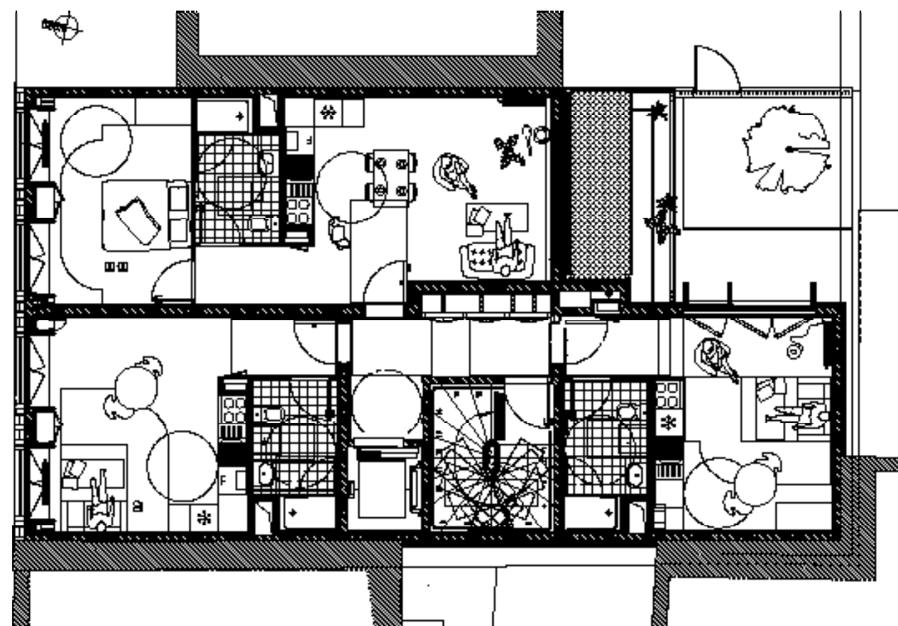
PLAN ÉTAGE COURANT
