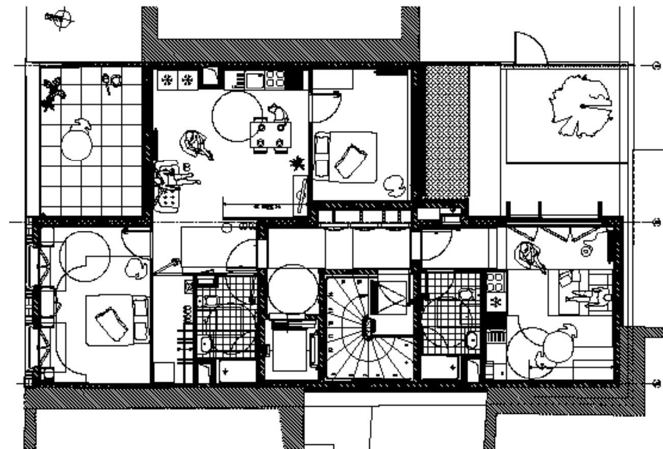
PLAN ÉTAGE COURANT
