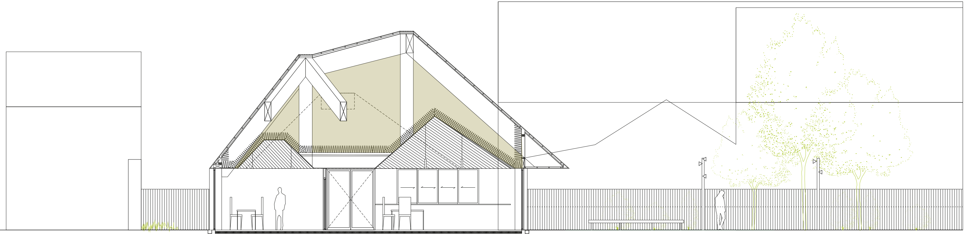
coupe AA'
